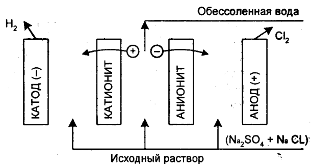
Рис. 4.6. Схема электродиализа
