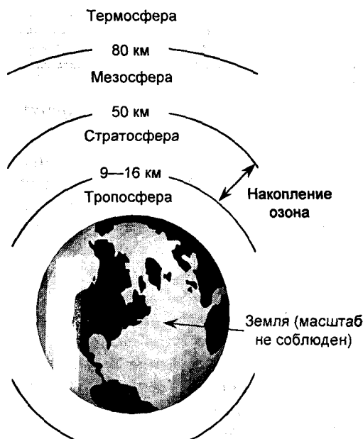
Рис. 4.3. Структура атмосферы
