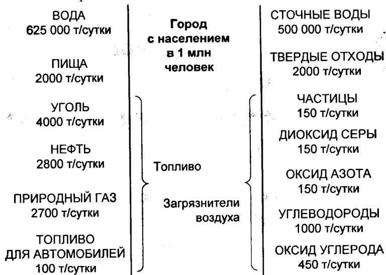
Рис. 4.1. Основные входные (вода, пища, топливо) и выходные (сточные воды, твердые отходы, загрязнители воздуха) потоки города
